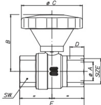
rozměry
