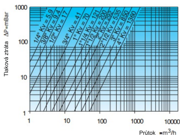
graf tlakové ztráty a průtoku
