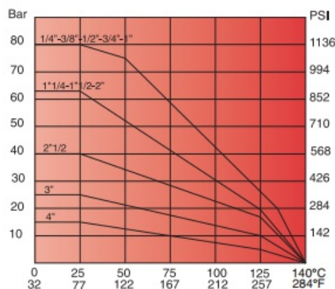
graf tlaku a teploty
