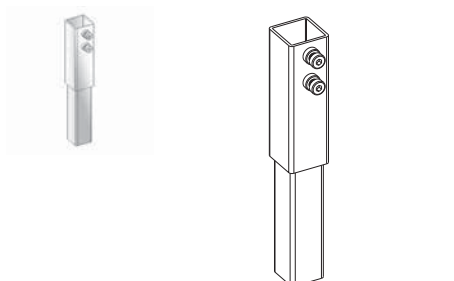
Nástavec stojánkových konzol RADIK a KORATHERM
